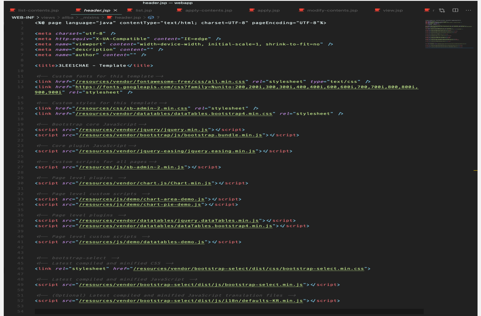
header.jsp
