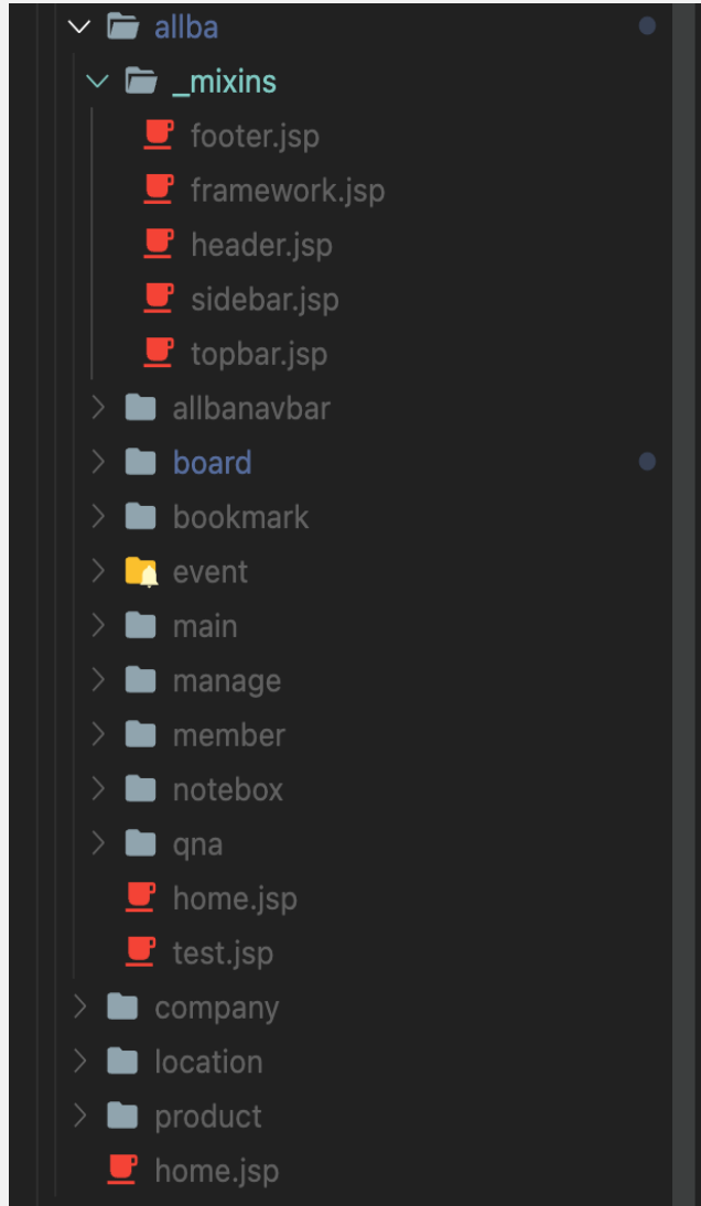
alba/_mixins 경로
